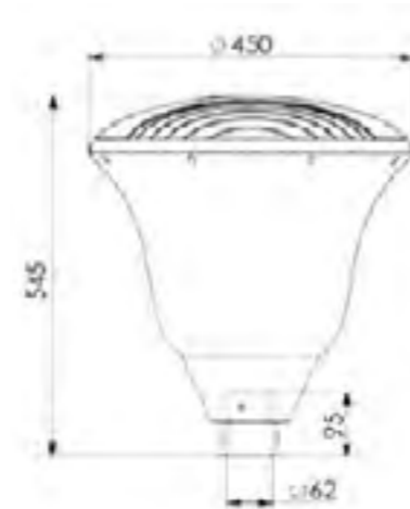
CASSIOPÉE 3000°K
